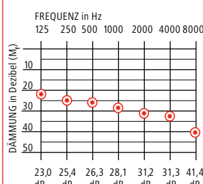
DLO®-Silikon DI-Filter Rot
